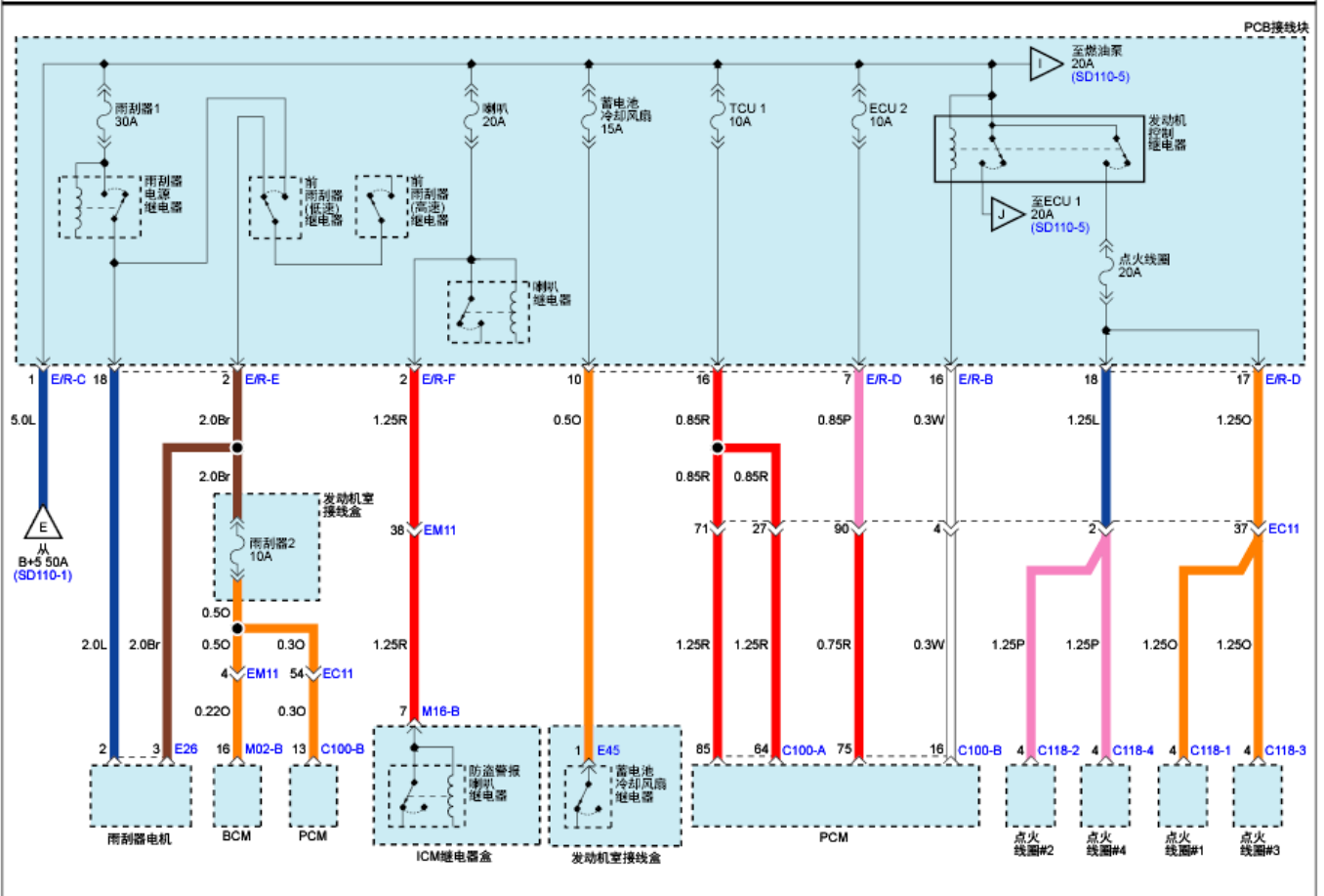
电源分布(4)
